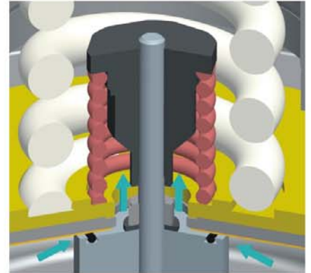
Válvula interna de alívio parcial Partial internal relief valve.
