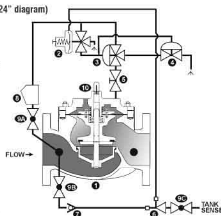
3333 (10-24" diagram)
